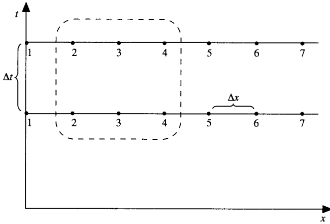
FIG. 4.8 An implicit finite-difference module.
